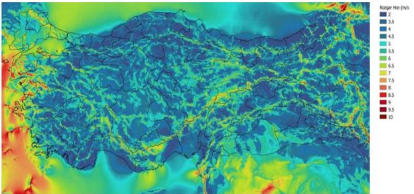
Harita: Türkiye Rüzgar Enerjisi Potansiyeli Atlası (2022)
